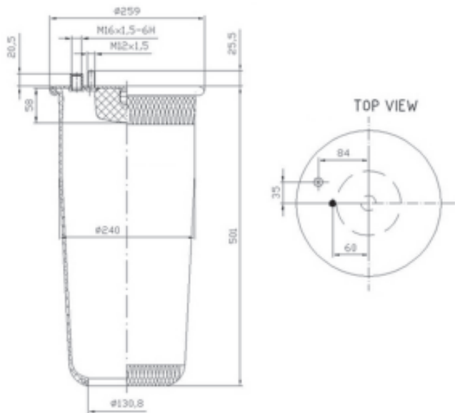
MAN 81.43601.0152
