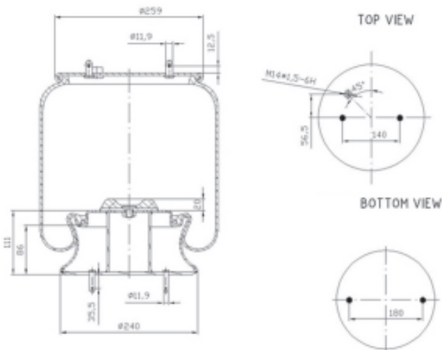
SCANIA 470920
